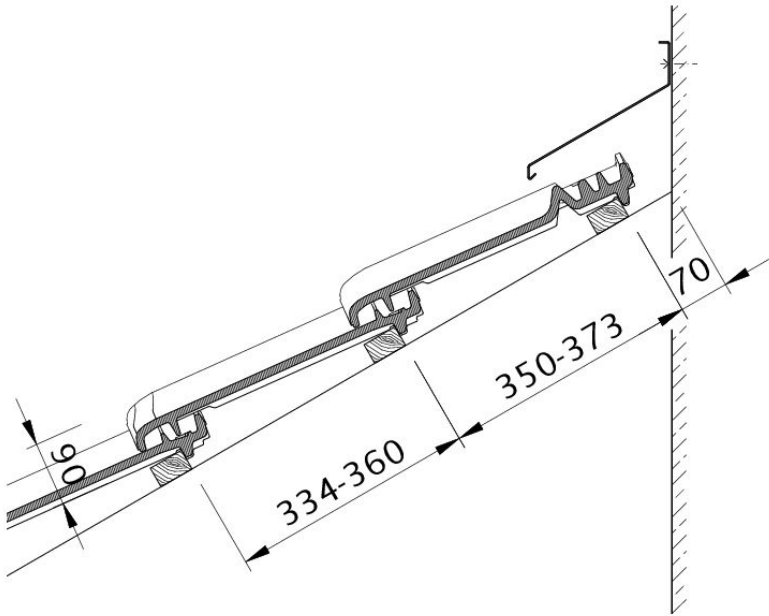
Desen tehnic produs MZ3 WMF WMF
