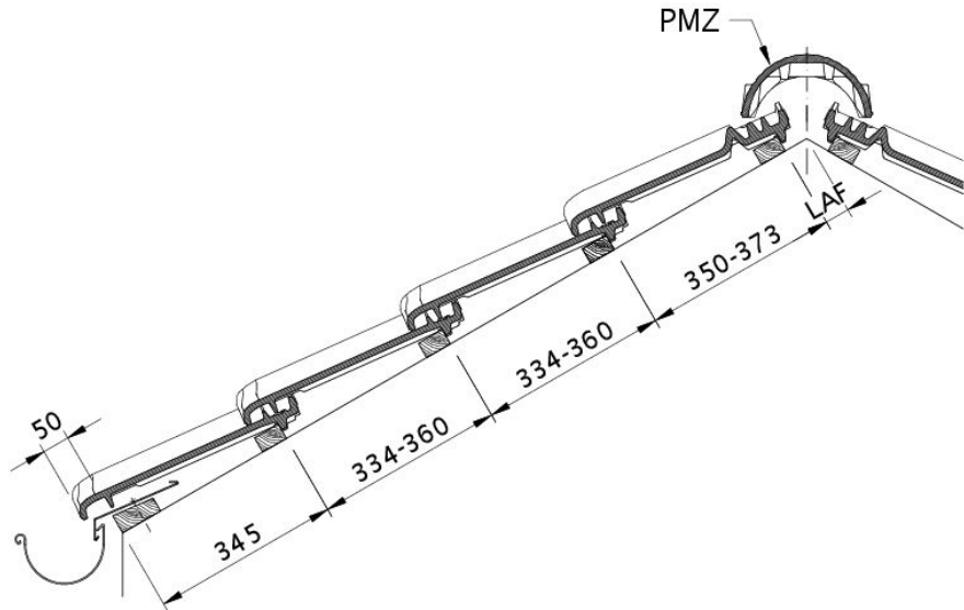
Desen tehnic produs MZ3 DQF DQF
