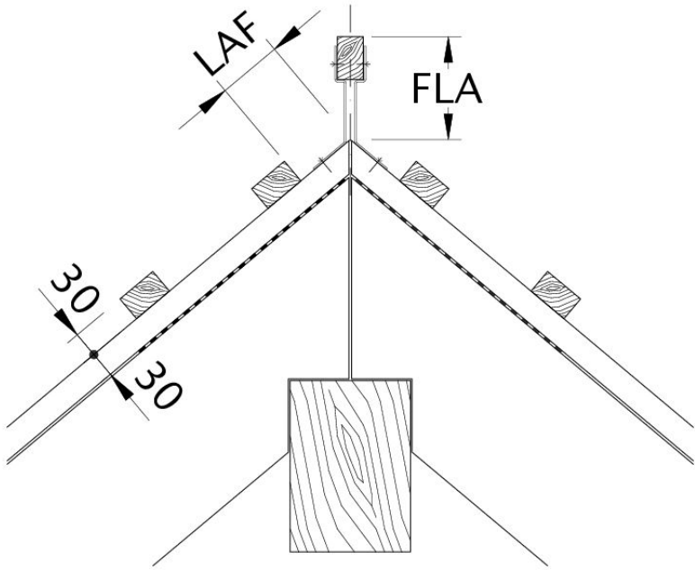
Desen tehnic produs KLASSIK DSC LAF
