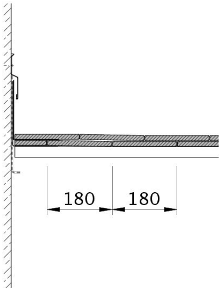
Desen tehnic produs KLASSIK WMF WMF-2
