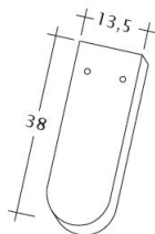
Desen tehnic produs KLASSIK 1-2
