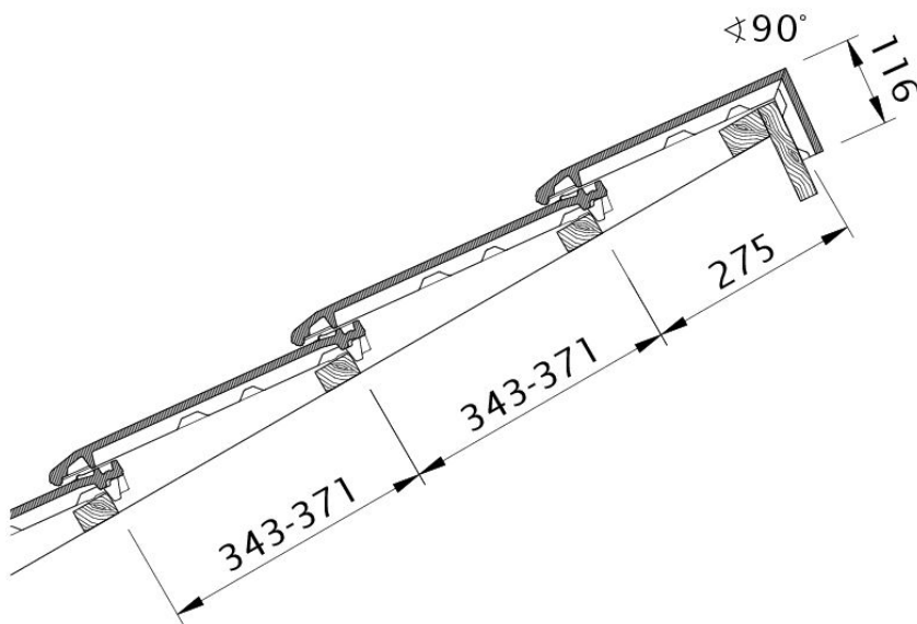
Desen tehnic produs MIKADO PDA PDA
