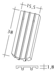
Desen tehnic produs PROFIL Kera-Saechs-15cm-AnAbfuehrer
